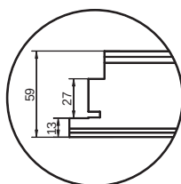
Przekrój skrzydła
